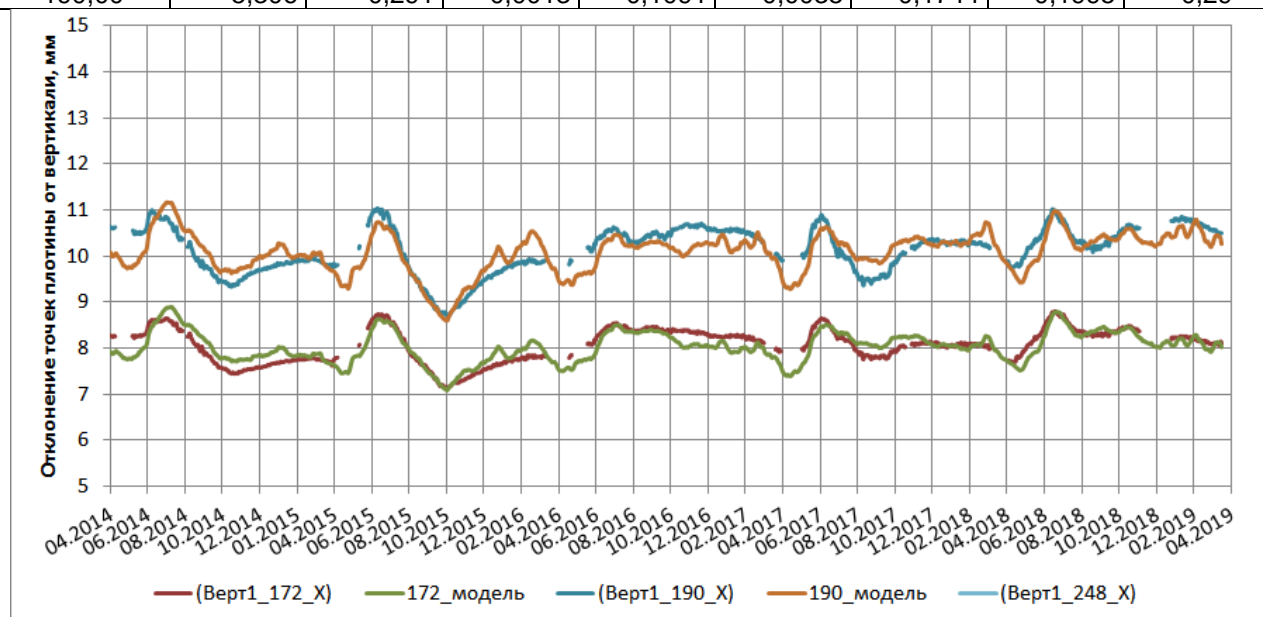
Рисунок Е.1 – Графики горизонтальных смещений стационарной секции гравитационной бетонной плотины, построенные по данным натуральных наблюдений по отвесам и полученные по прогнозным регрессионным моделям
